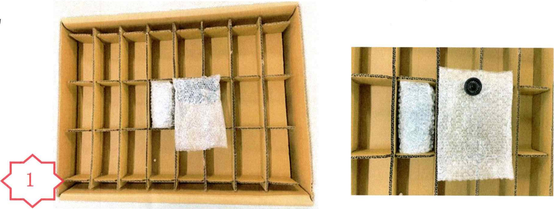
图一，每 10 个组件用一个小气泡袋装，每格 2 袋，每格 20pcs，每层 24 格，每层 480pcs，共 3 层，满箱 1440pcs
